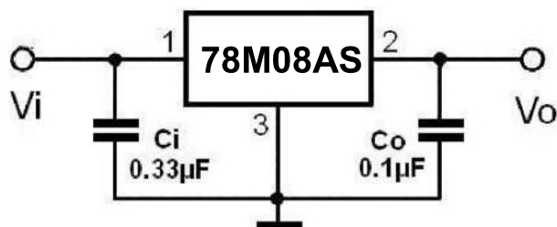
Figure.1 DC Parameter
